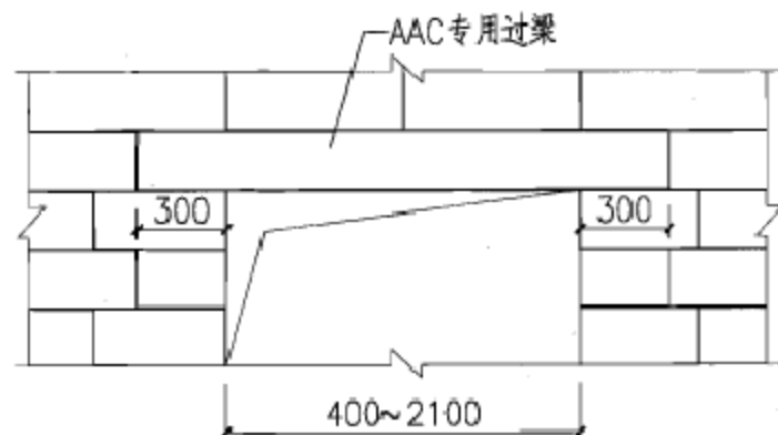
单个门窗洞口过梁
