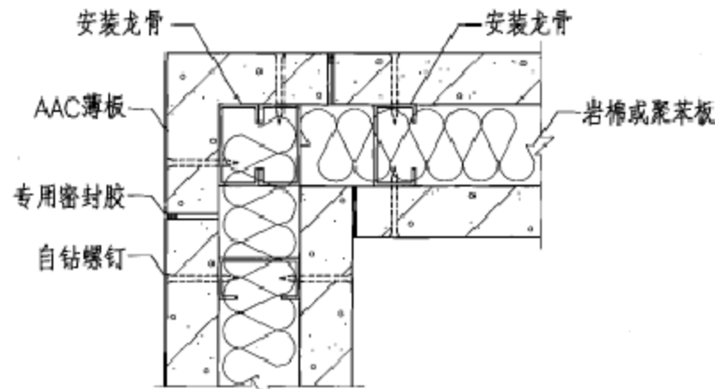
3 采用转角板
