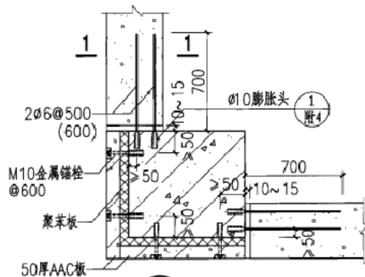
1 拉结筋连接
