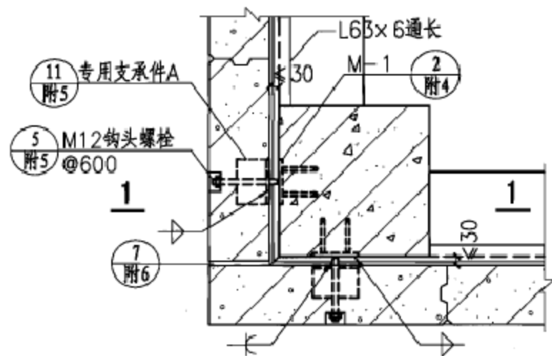
1 钩头螺栓法
