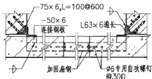
2-2 (混凝土结构)
