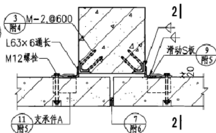
3 滑动螺栓法
