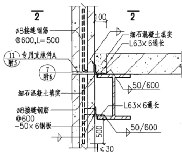
2 插入钢筋法
