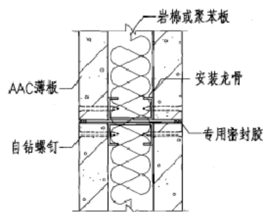
1-1 (板缝)
