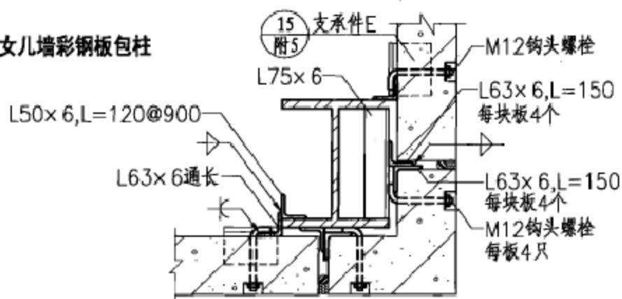
4 转角板安装
