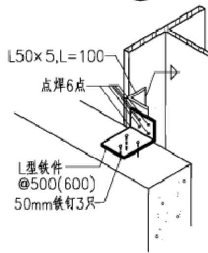
透视图
