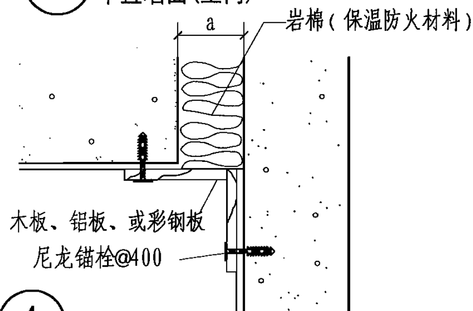
3 平直墙面(室内)
