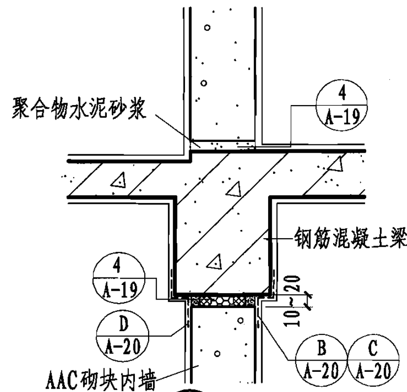
6 卫生间隔墙 (二)
