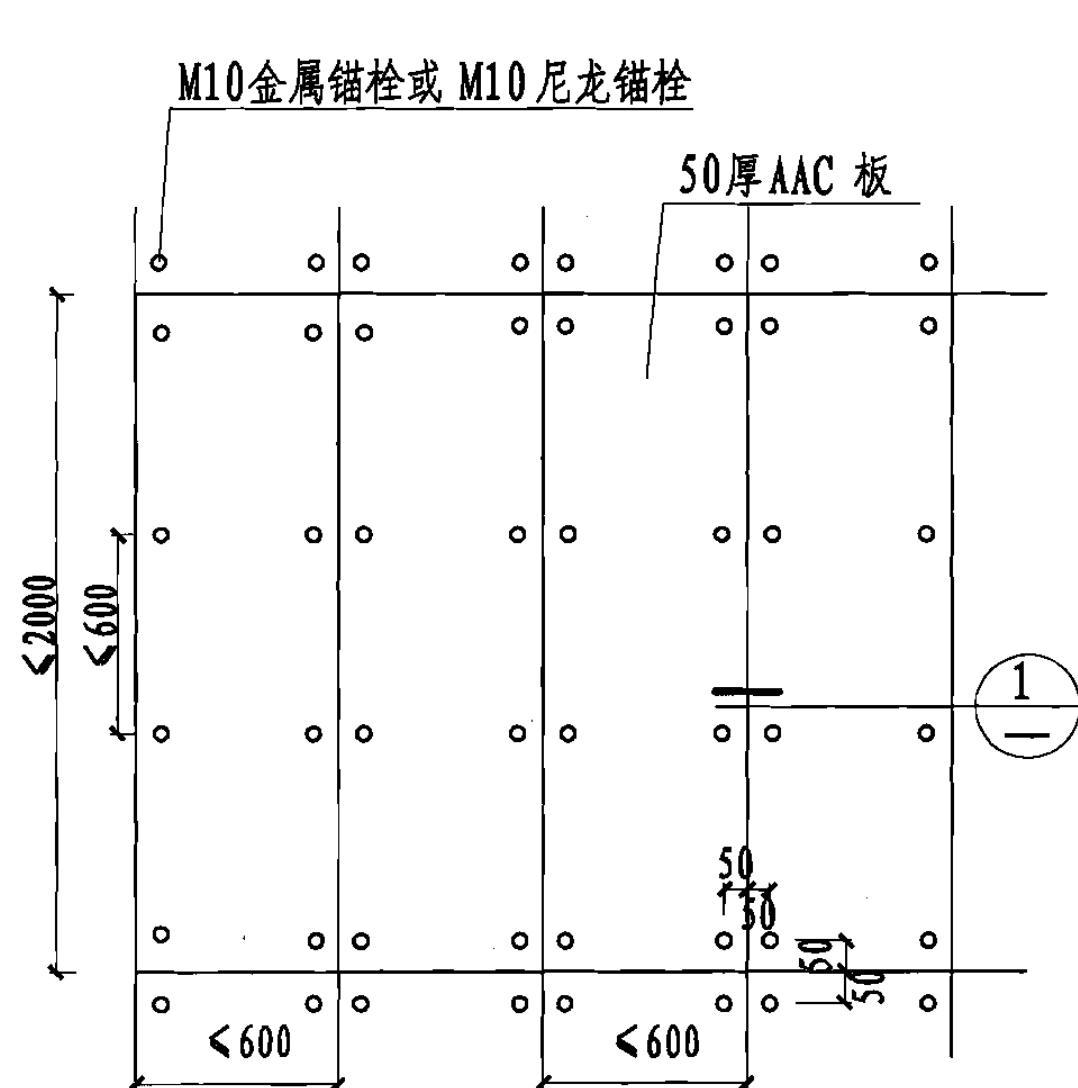
竖板保温立面
