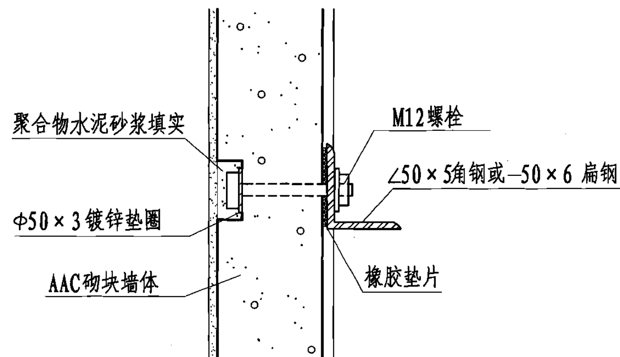
2 金属支架安装示意
