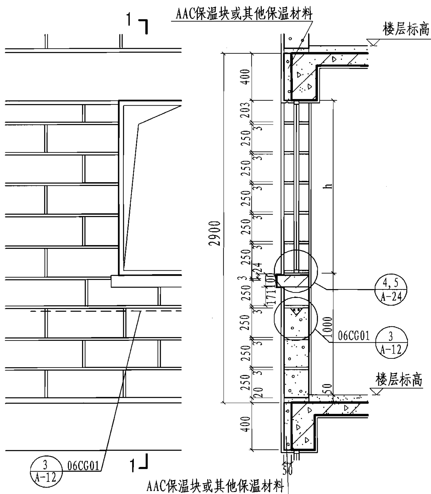
1000高窗台砌块排列示意
