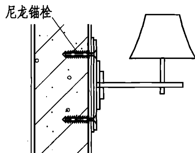
轻便重物安装 (10kg以下)
