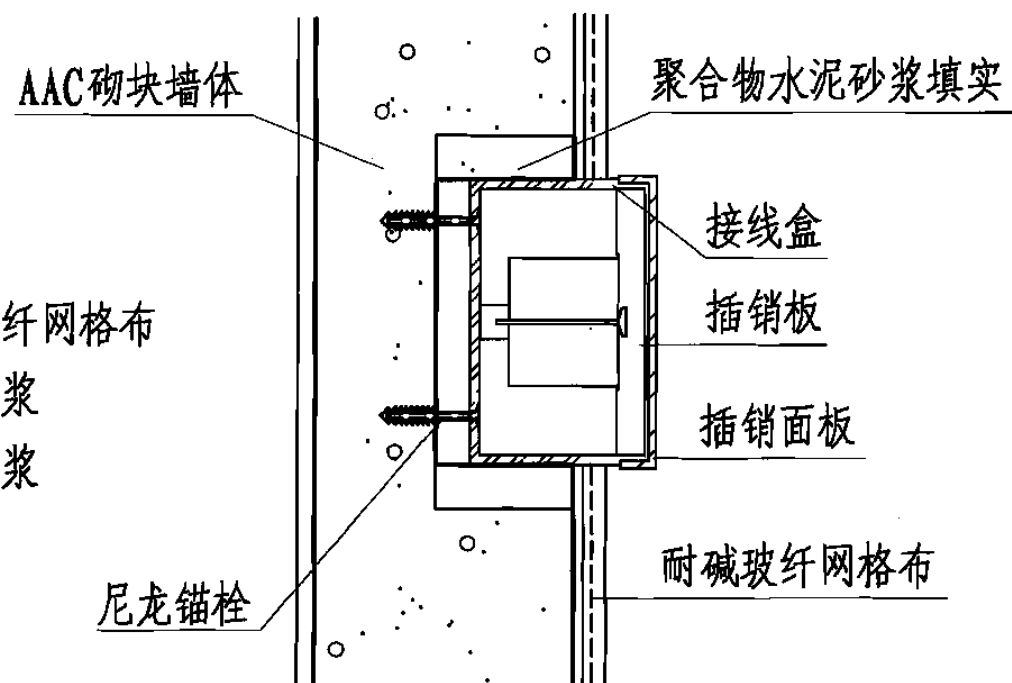
4 插销(或接线盒)安装示意
