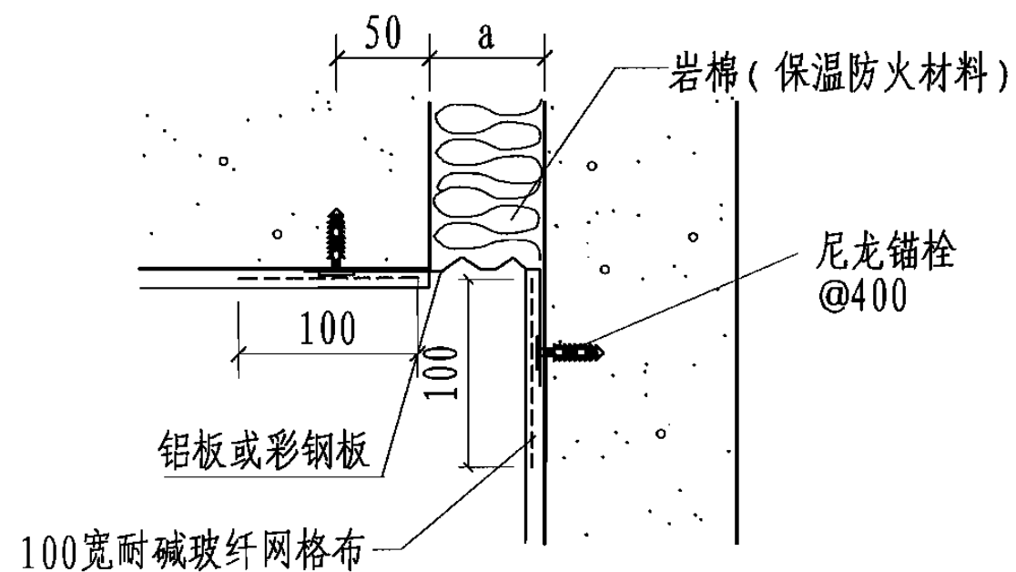
1 L型墙面(室外)
