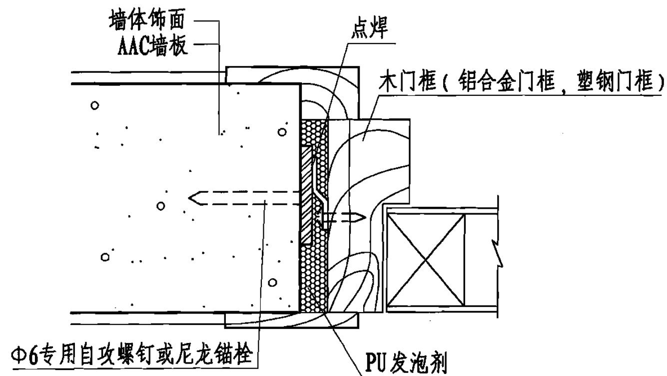
3 扁钢加固
