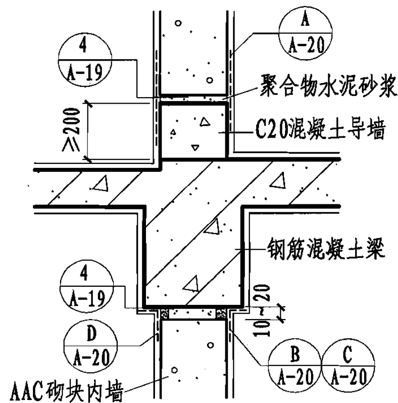
5 卫生间隔墙 (一)
