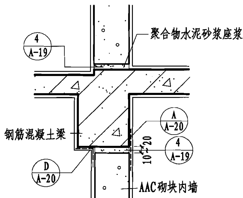
5 卫生间隔墙 (一)
