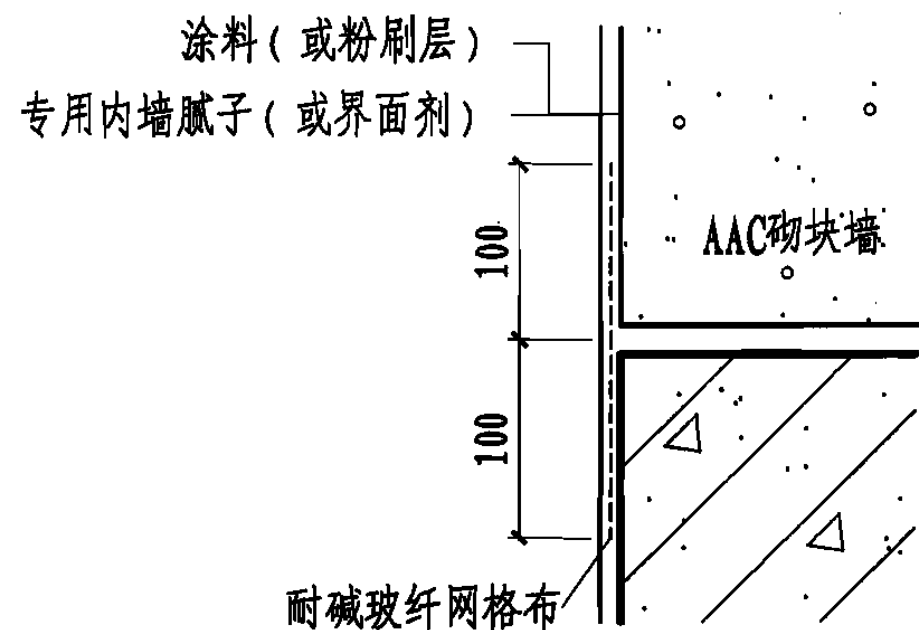
A 接缝防裂措施
