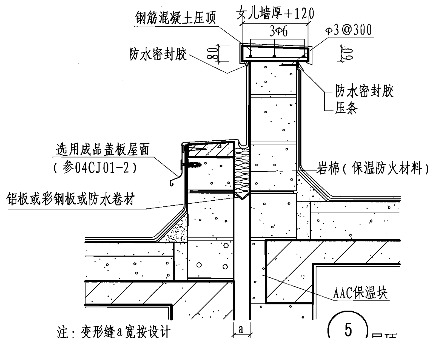
2 平直墙面(室外)
