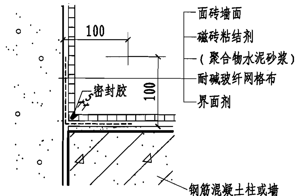
D 阴角防裂措施 (三)
