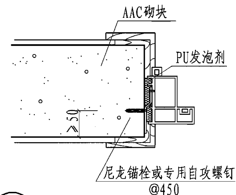
6 塑料门框 (铝合金门框)
