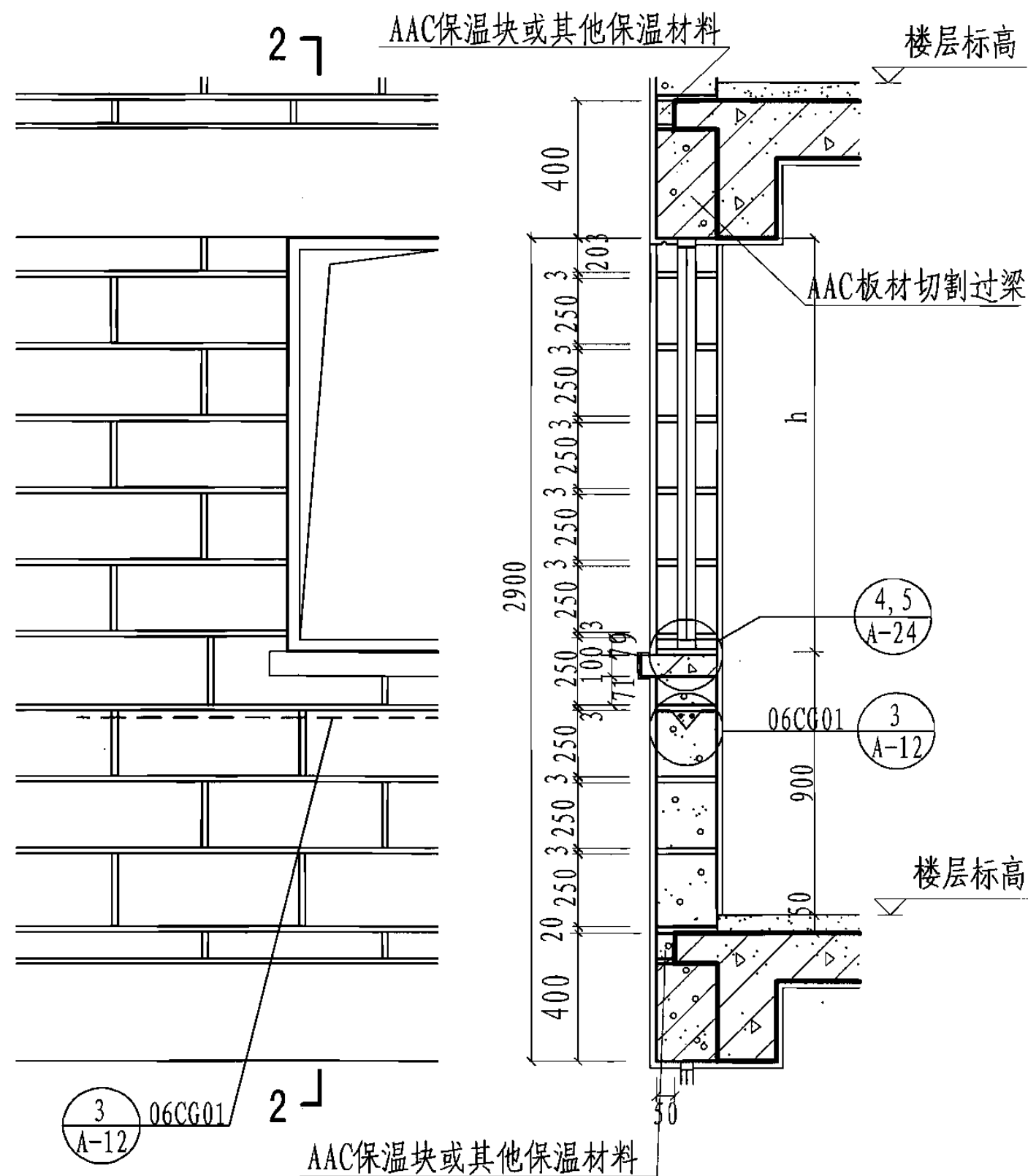
900高窗台砌块排列示意
