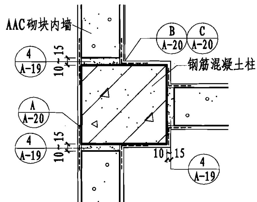
1 一般钢筋混凝土结构
