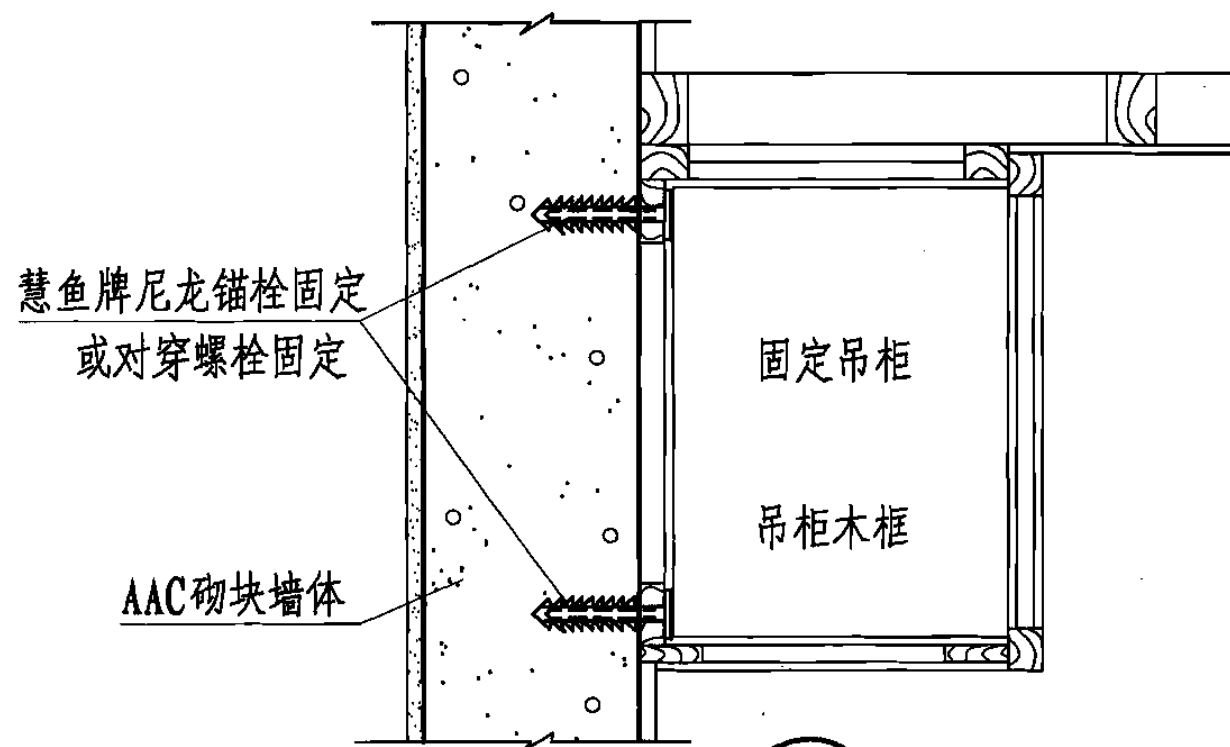
1 吊柜安装示意
