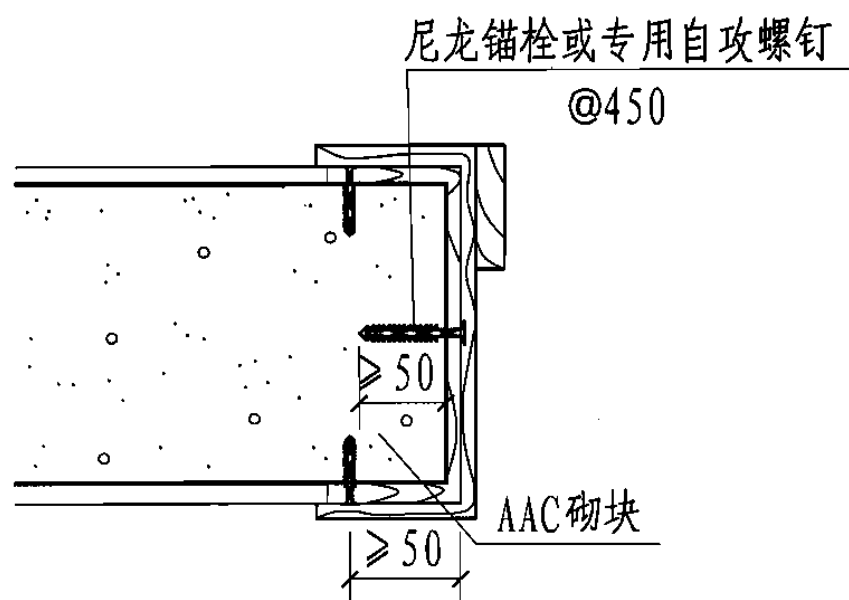
4 装饰木门框
