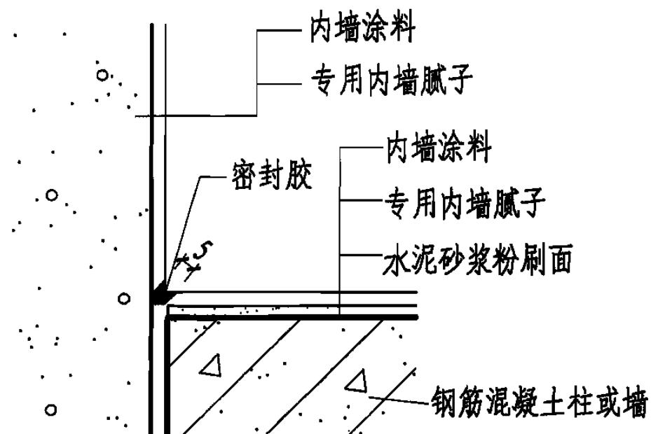
C 阴角防裂措施 (二)
