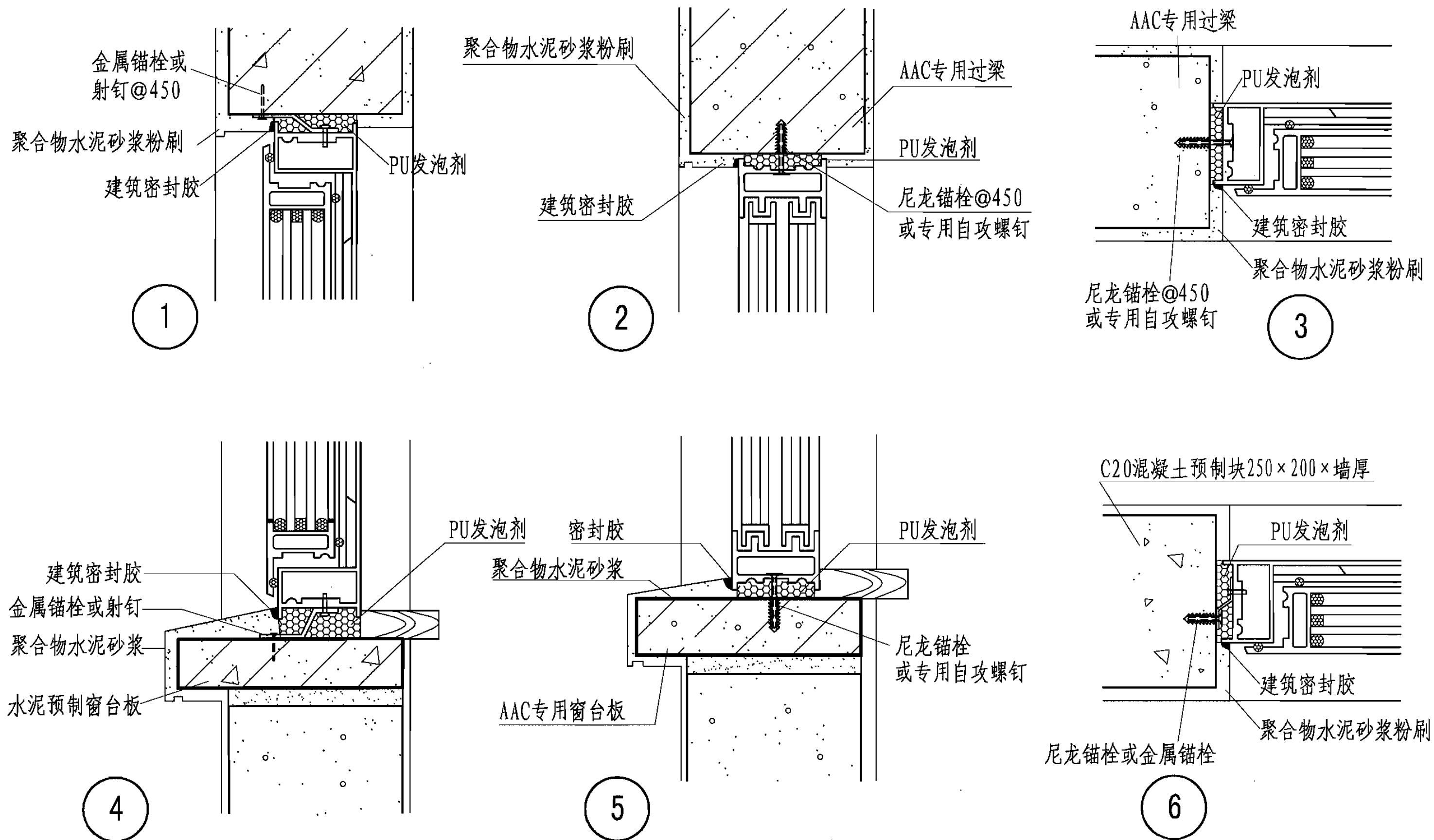
窗安装节点图
