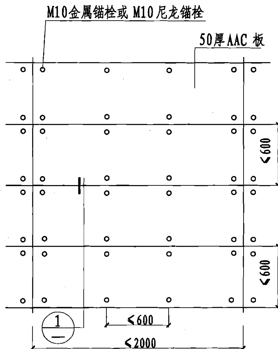
横板保温立面
