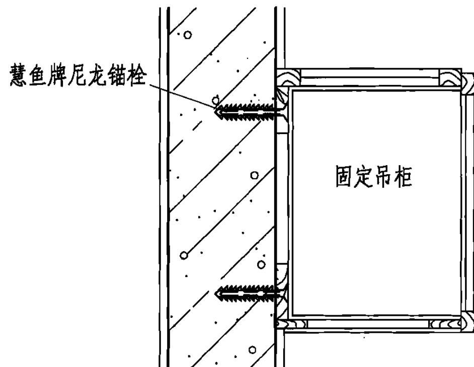
吊柜安装
