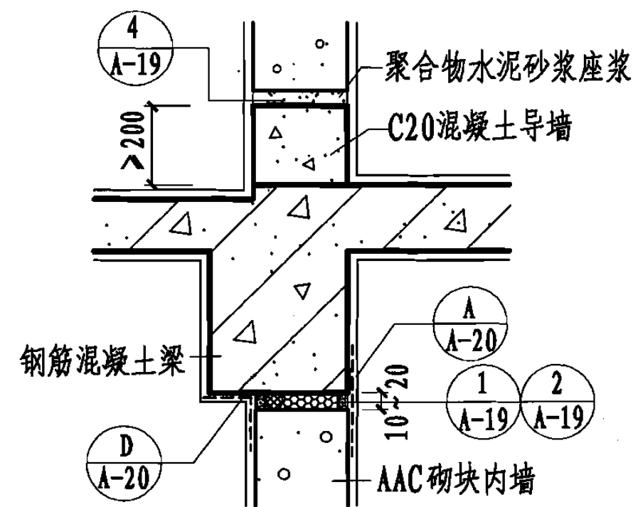
6 卫生间隔墙 (二)
