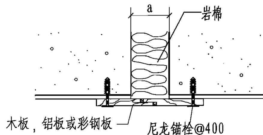
3 平直墙面(室内)
