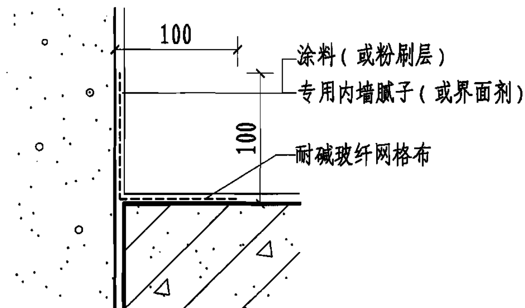
B 阴角防裂措施 (一)
